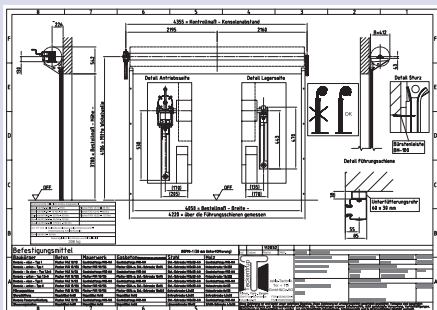
Jedem Rolltor liegt neben der Montageanleitung eine individuelle, auftragsbezogene Montagezeichnung bei.
