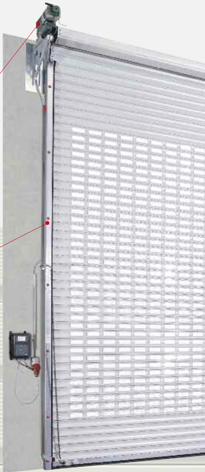
Die Fangvorrichtung verhindert im Notfall den Absturz des Torbehanges.
