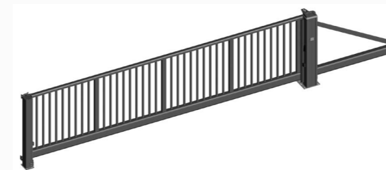
Schiebetor B.ALU CLASSIC Schrägbau Breite max. 15 m freitragend Höhe max. 2,5 m
