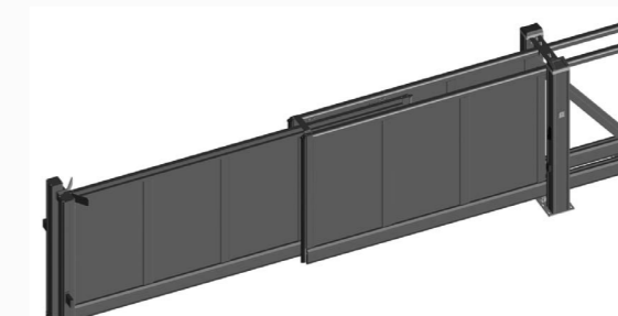
B.ALU Teleskopschiebetor Breite max. 21 m freitragend Höhe max. 2,5 m
