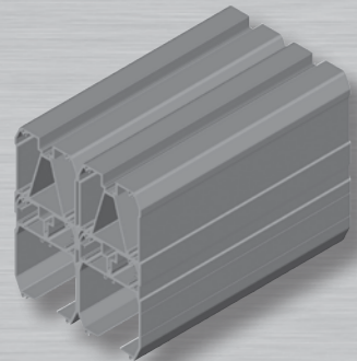
Doppelschiebetorprofil HST 3/7/2 300 x 350 mm selbsttragendes Aluminiumprofil für Tore bis 25 m Pfostenlichte
