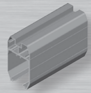
Schiebetorprofil HST 4 117 x 200 mm selbsttragendes Aluminiumprofil für Tore bis 7 m Pfostenlichte
