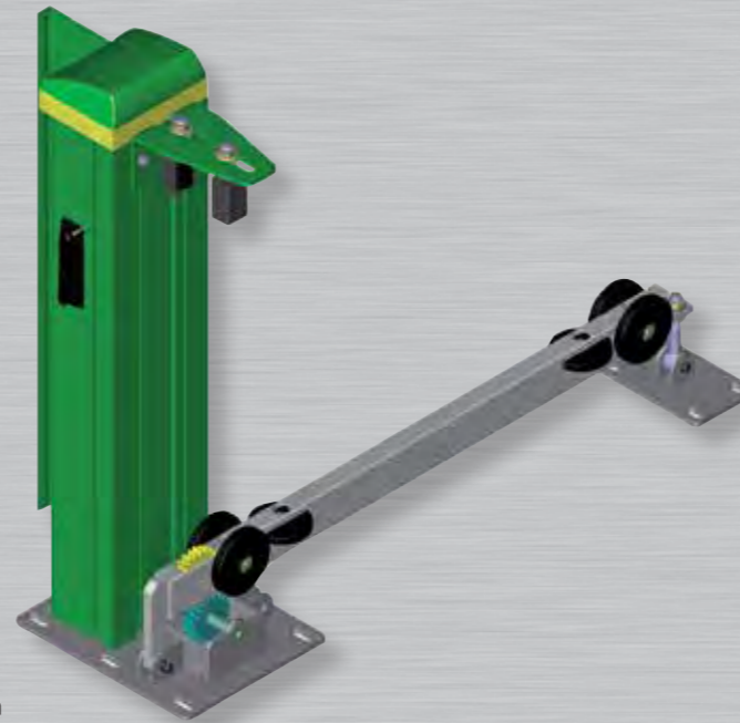
Rahmenprofil HST 9 100 x 100 mm für Schiebetore bis 16 m Drehtore bis 10 m
